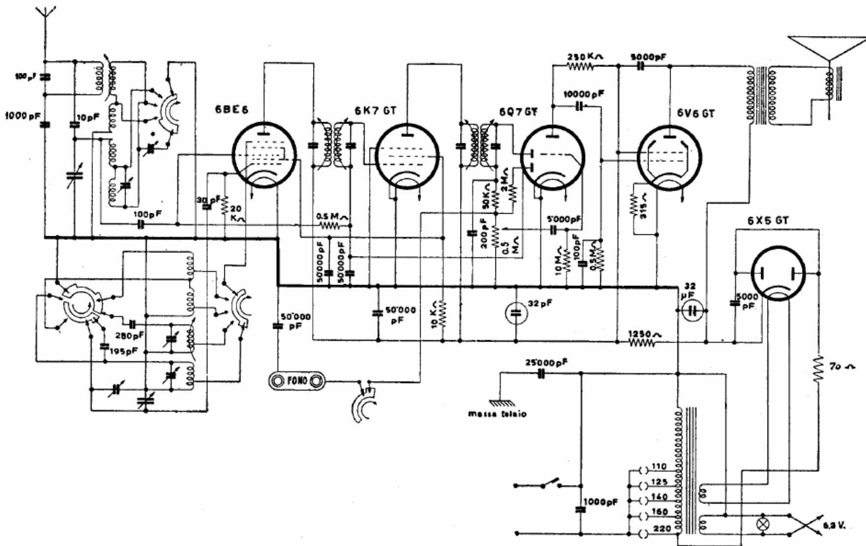
IRRADIO - Modd. AK 14 e AK 15 - Media frequenza 467 kc. Potenza d'uscita 3 watt. Consumo 40 watt.
